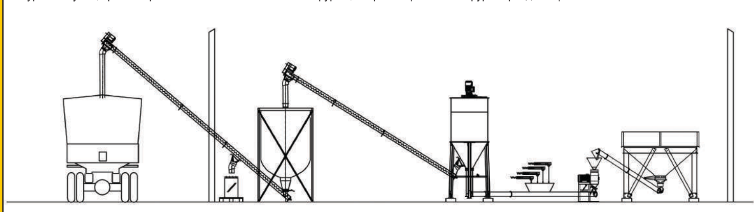
Фуражна кухня, транспортна техника към силос за готов фураж, изпразващ шнек към фуражораздаващо
