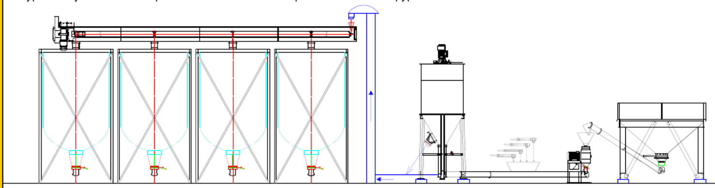
Фуражна кухня с елеватор и външни силози за съхранение на готов фураж
